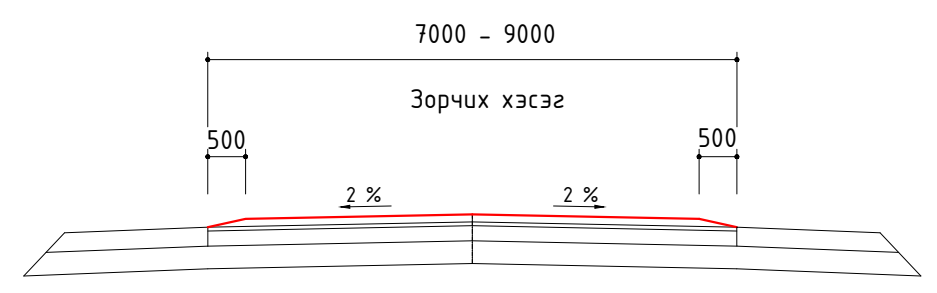
ХӨНДЛӨН ОГТЛОЛЫН ЗУРАГ А-А ОГТЛОЛ
